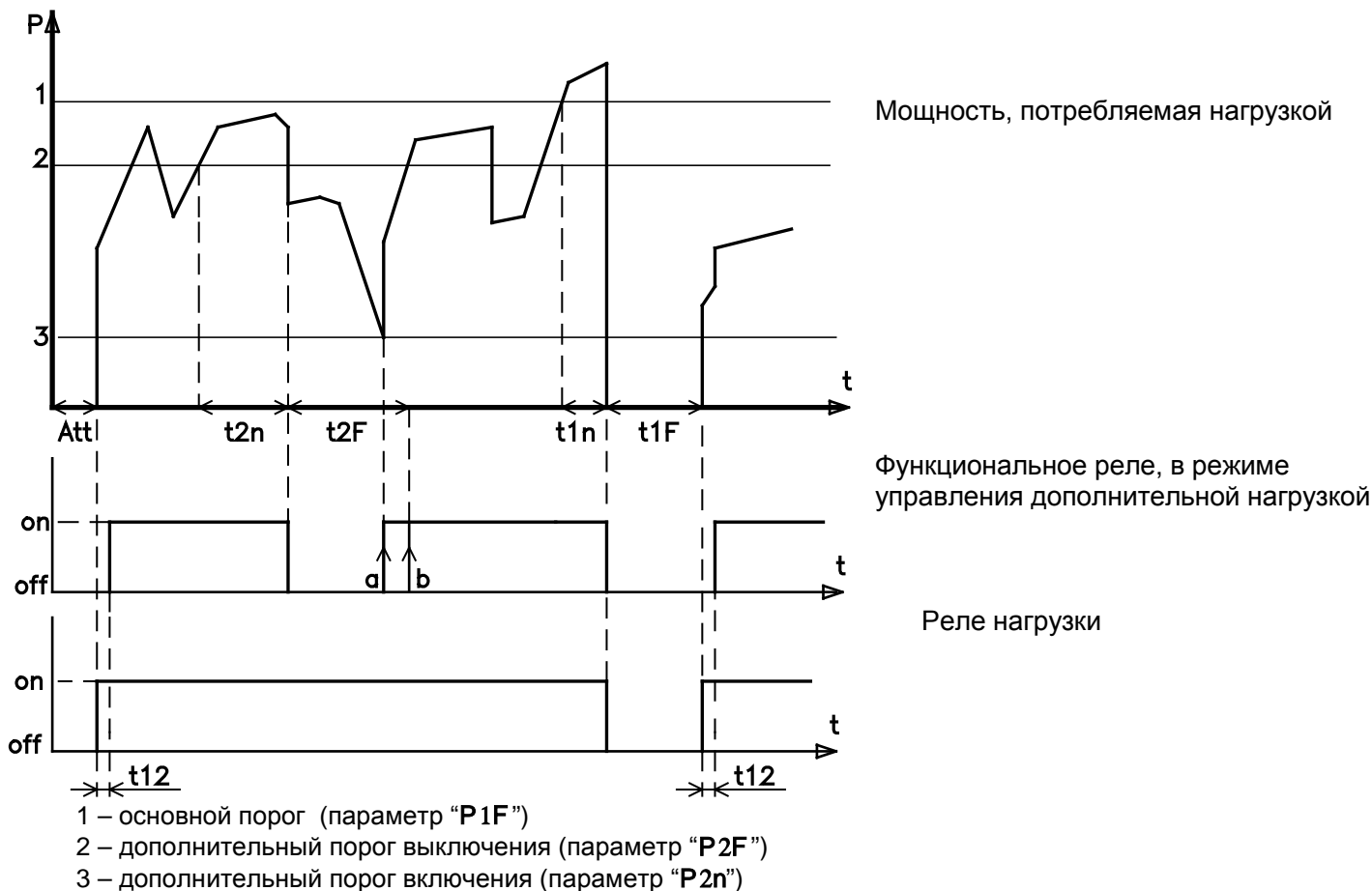
Рисунок 1.3 - Работа ОМ-310 в режиме ограничения мощности при r r S=2
