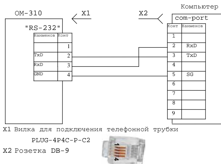
Рисунок 2.2 - Схема подключения ОМ-310 к компьютеру
